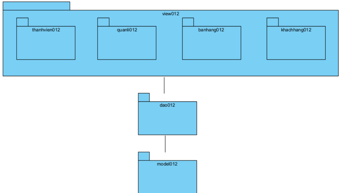
Biểu đồ gói cho toàn hệ thống
