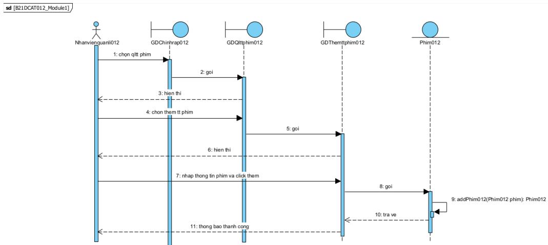
Biểu đồ tuần tự pha phân tích cho module 1
