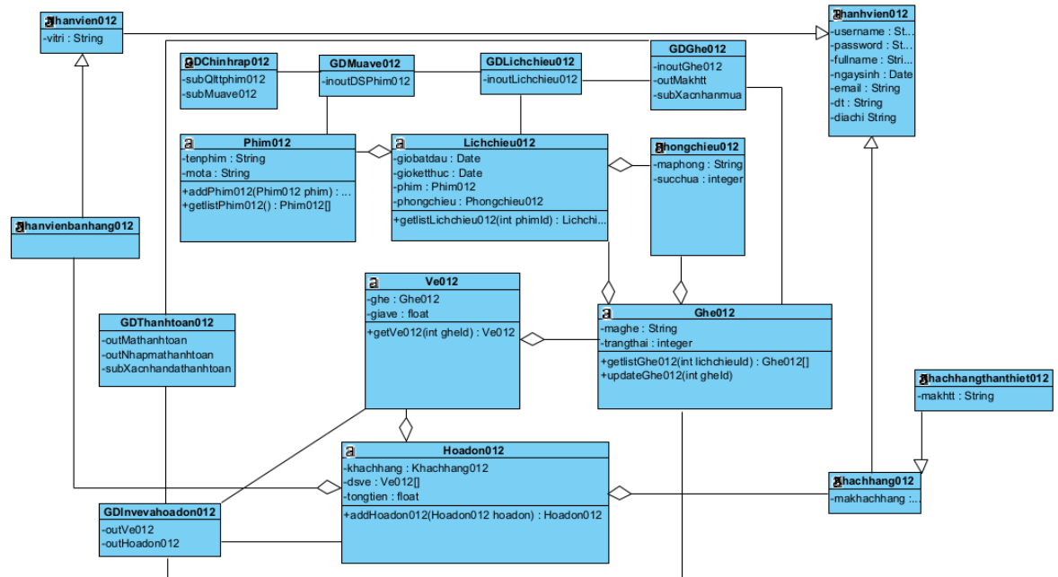
Biểu đồ lớp cho module 2
