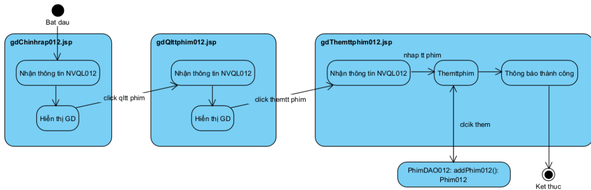
Biểu đồ hoạt động module 1
