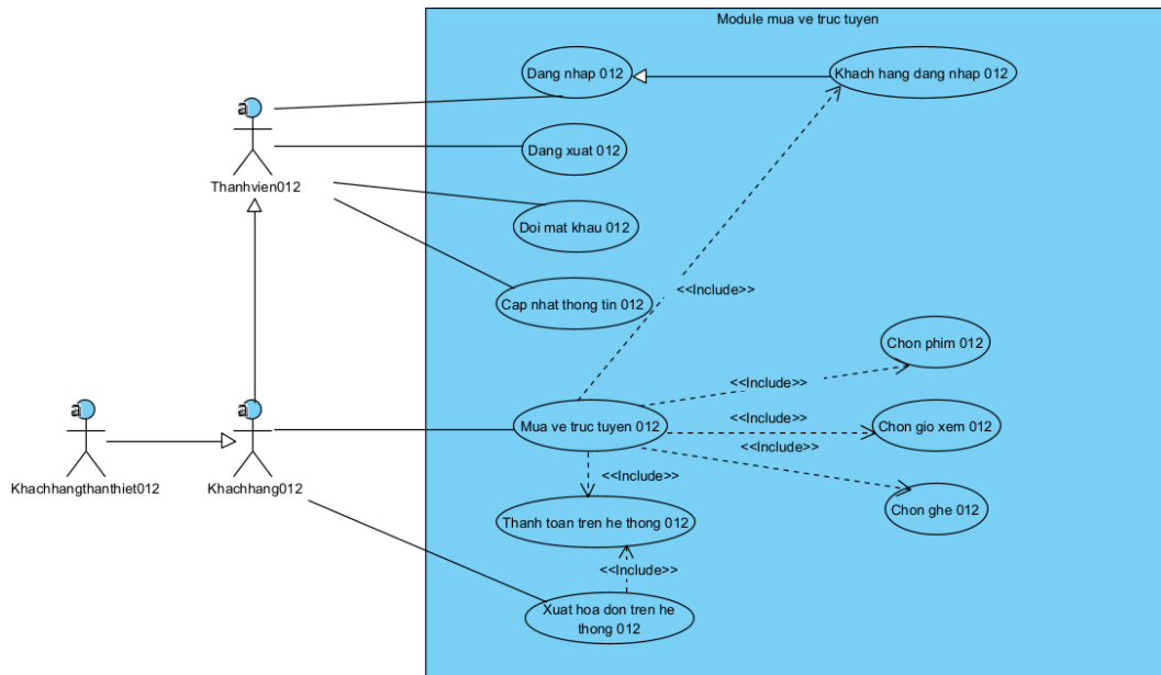
Biểu đồ usecase module 2
