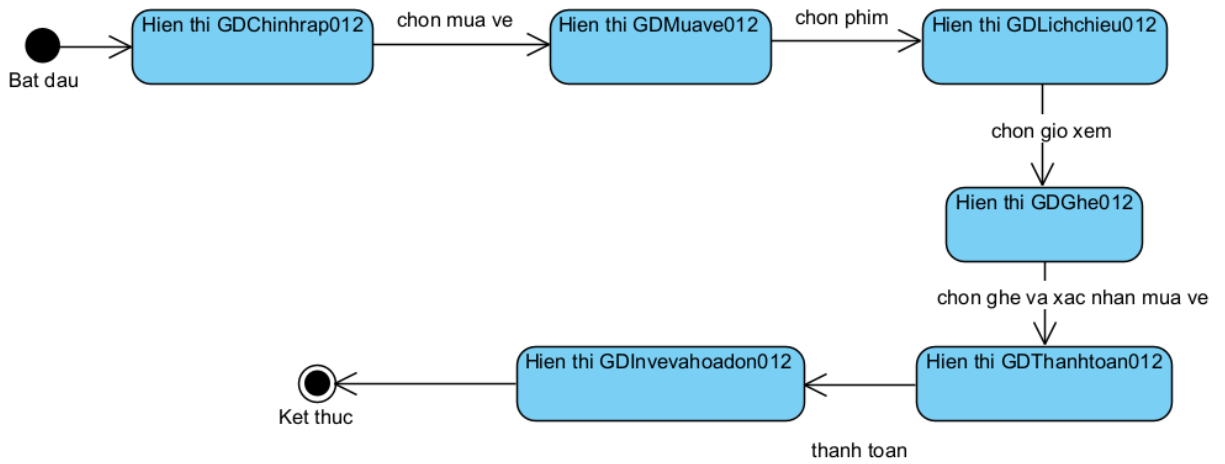
Biểu đồ trạng thái cho module 2
