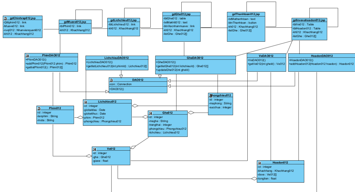
Biểu đồ lớp module 2
