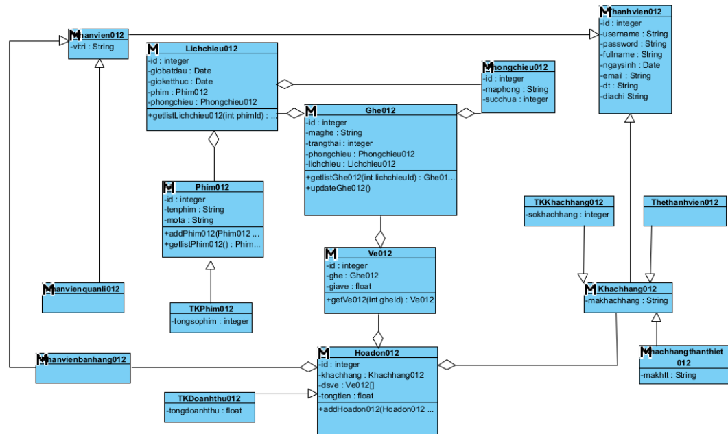
Biểu đồ lớp cho toàn hệ thống
