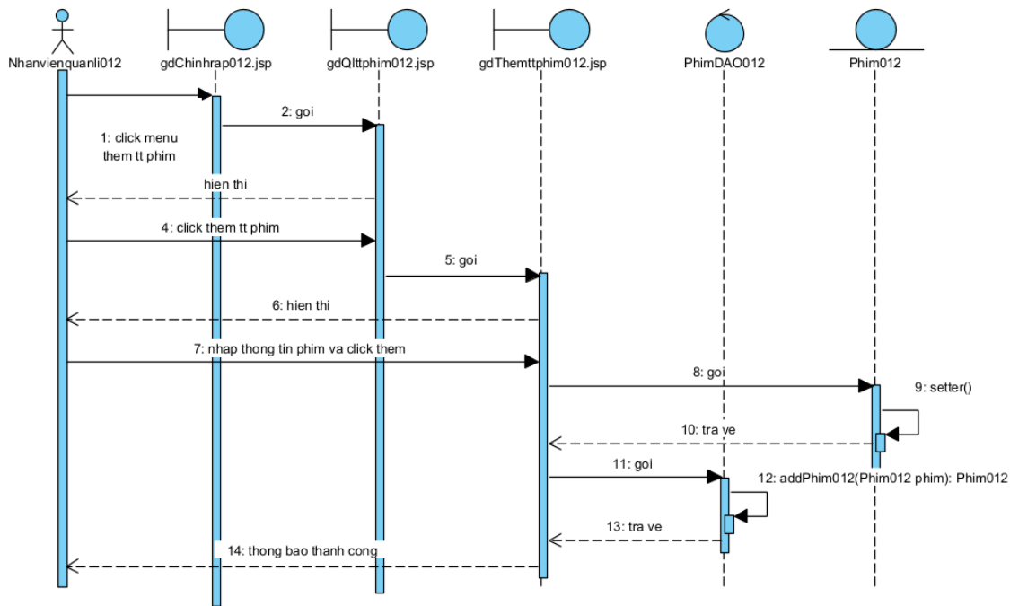
Biểu đồ tuần tự module 1
