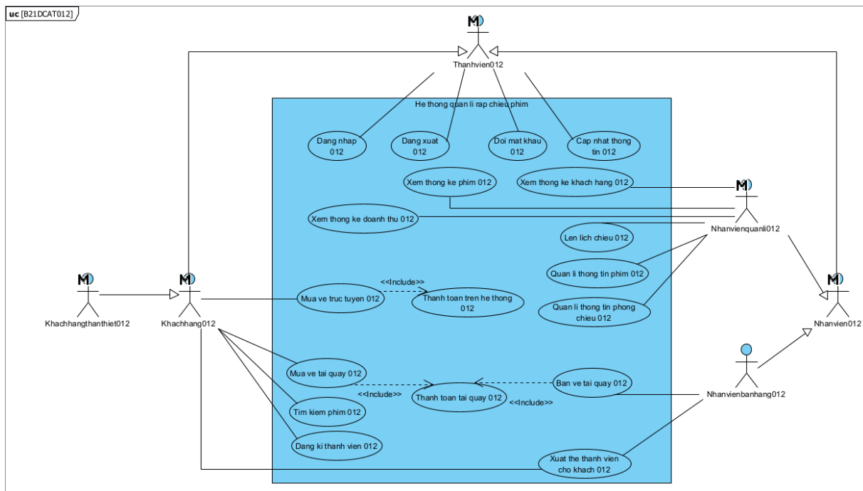
Biểu đồ usecase tổng quan
