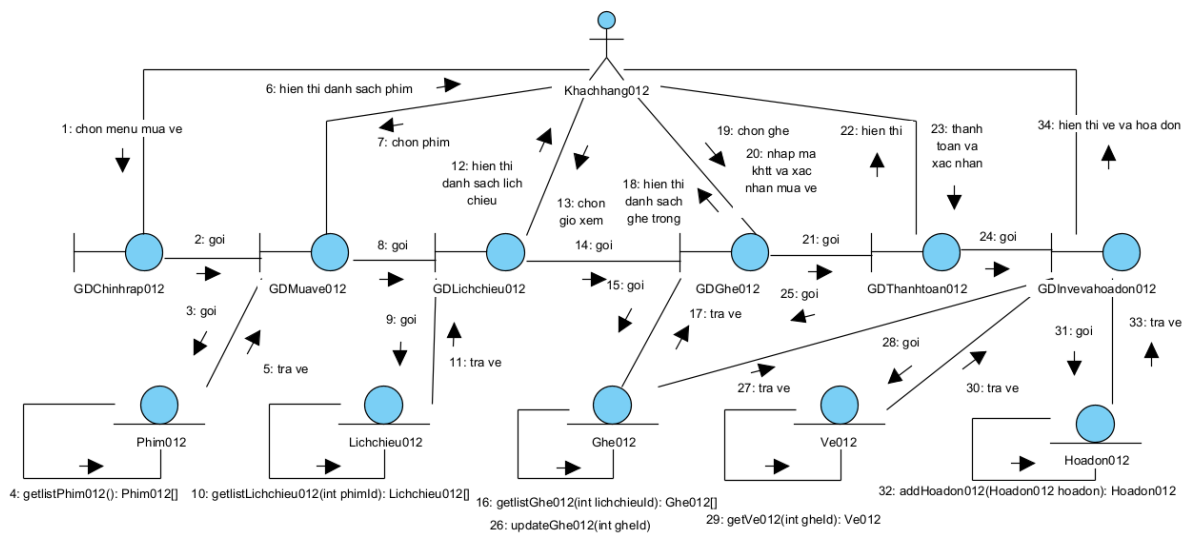
Biểu đồ giao tiếp cho module 2
