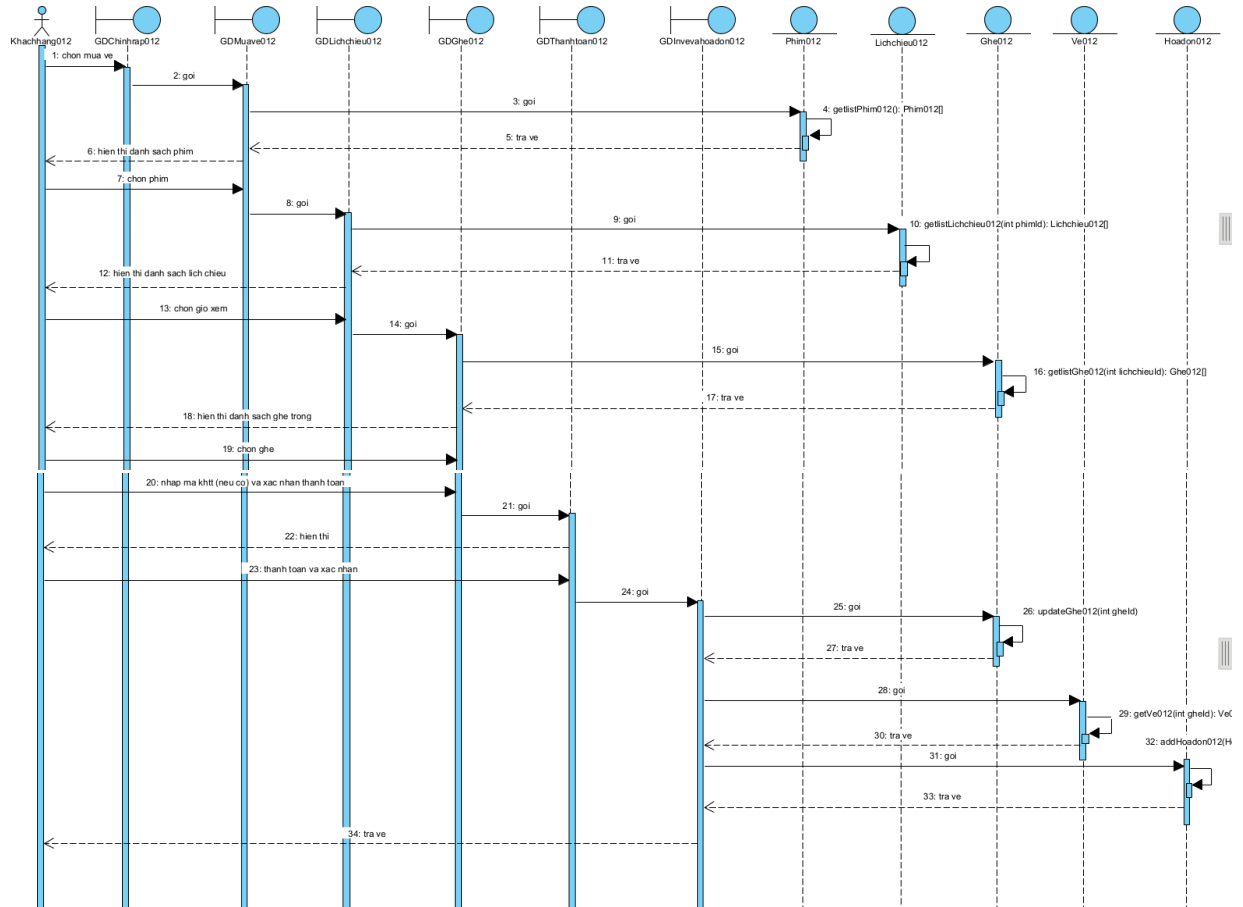
Biểu đồ tuần tự pha phân tích cho module 2
