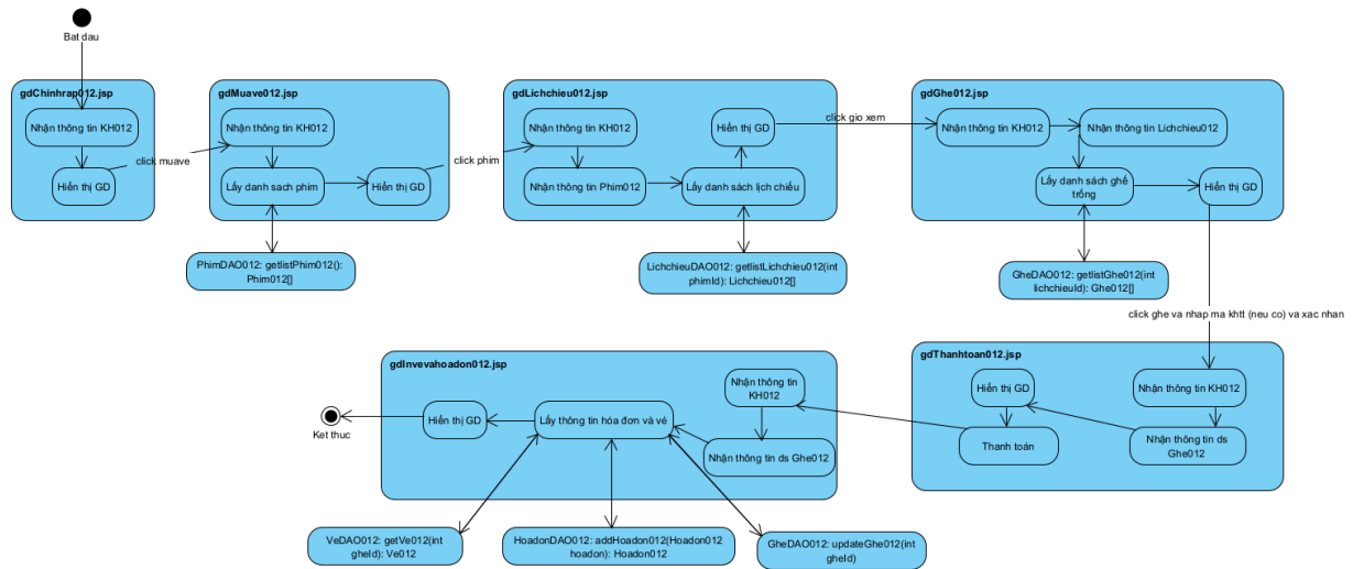
Biểu đồ hoạt động module 2
