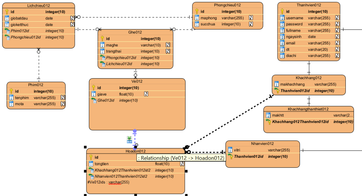
Cơ sở dữ liệu cho toàn hệ thống
