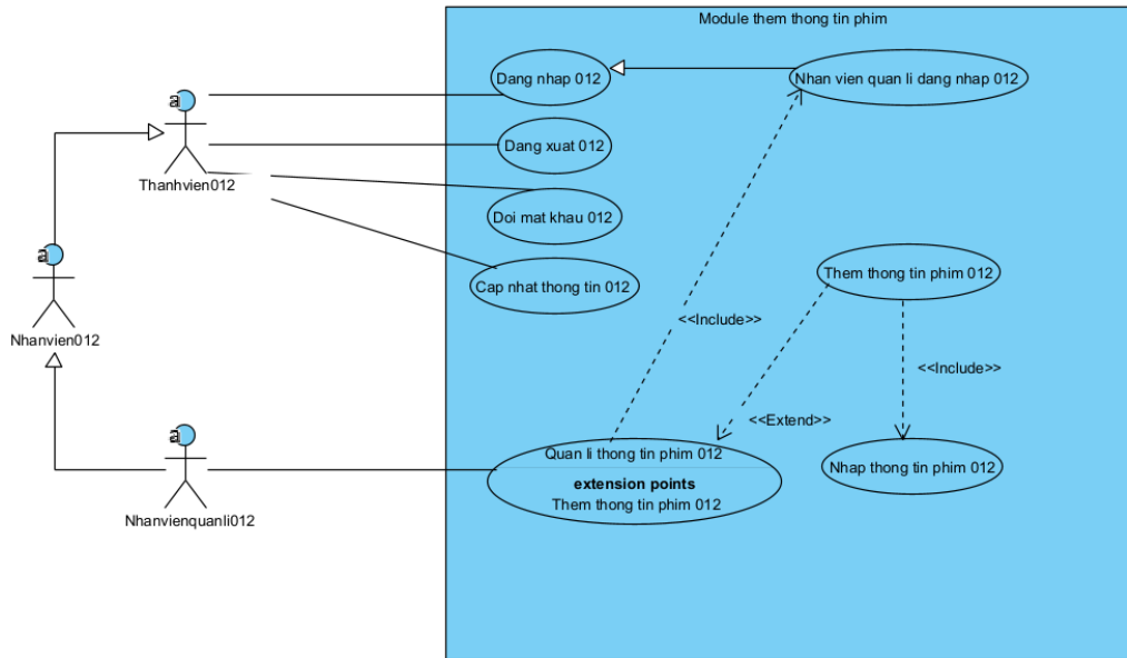
Biểu đồ usecase module 1
