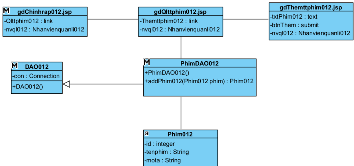
Biểu đồ lớp module 1
