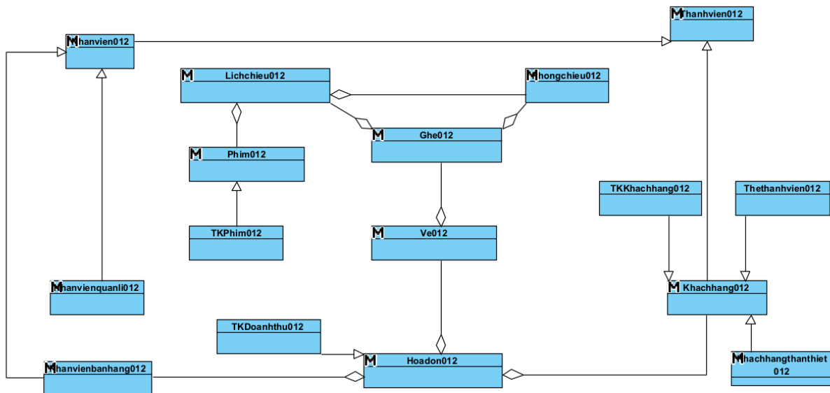
Biểu đồ lớp thực thể của hệ thống
